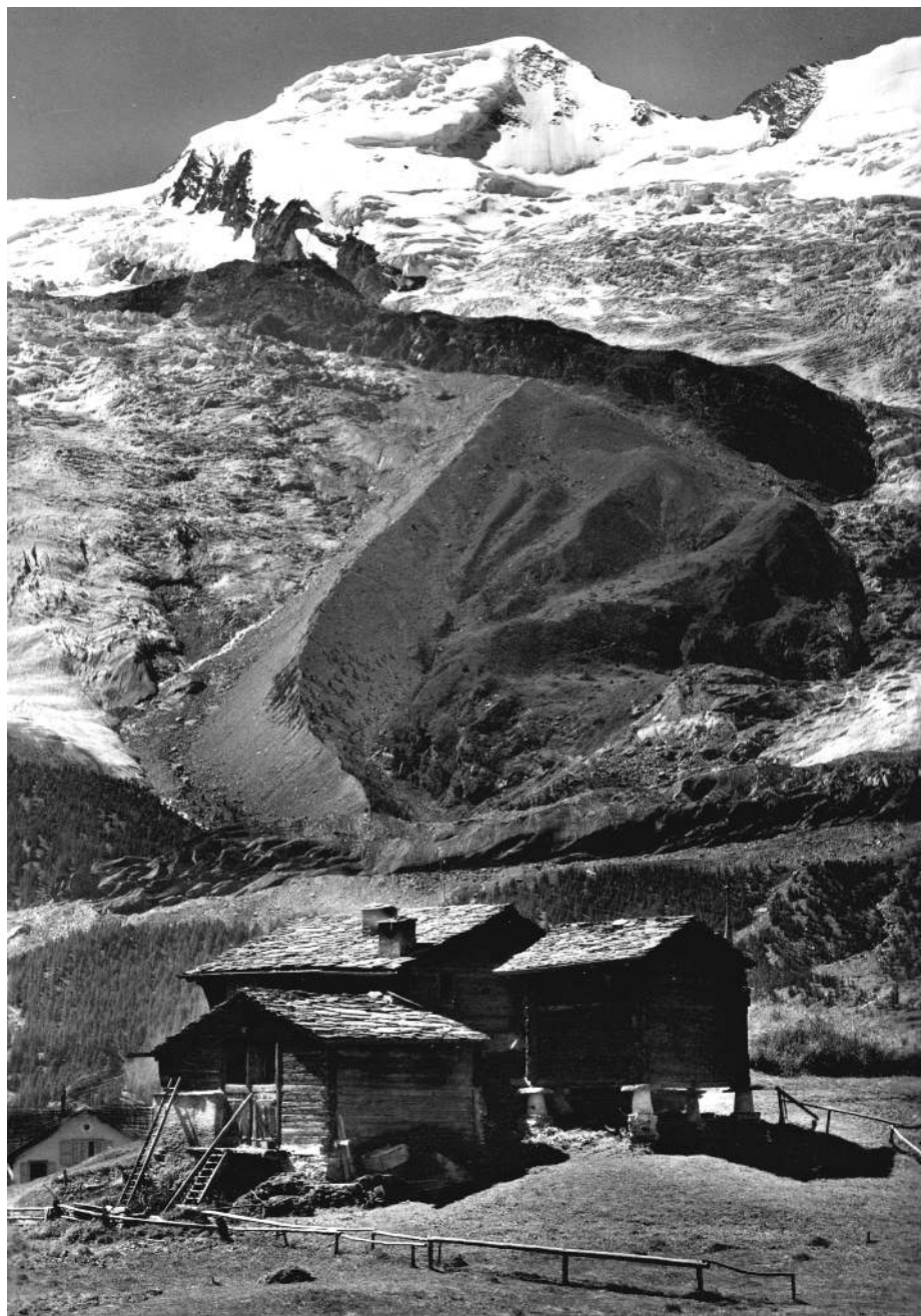
Gletscheralp - Alphubel, Saas-Fee (Foto: Gyger & Klopfenstein, Adelboden; Bildarchiv Georg Jäger).
